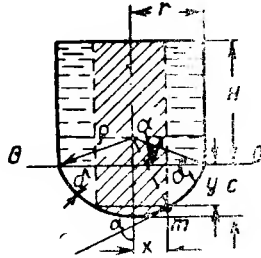
Рис. 17.13. Расчетная схема для определения безмоментных напряжений в сферическом днище сосуда, загруженного гидростатическим давлением
