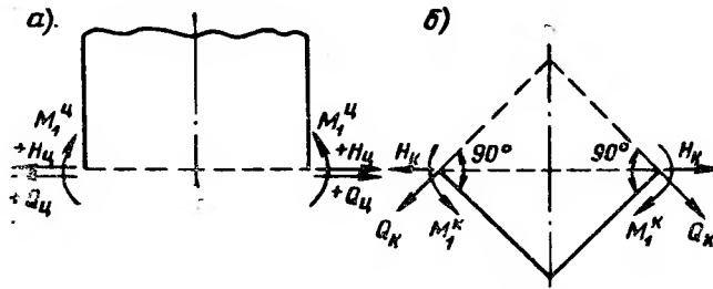
Рис. 19.15. Положительные направления усилий в сечениях оболочек
