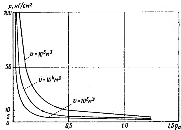
Рис. 21.5. Значение коэффициента \eta_a = \frac{a_r}{a_{ж}} при различных давлениях и объемах шаровых резервуаров
