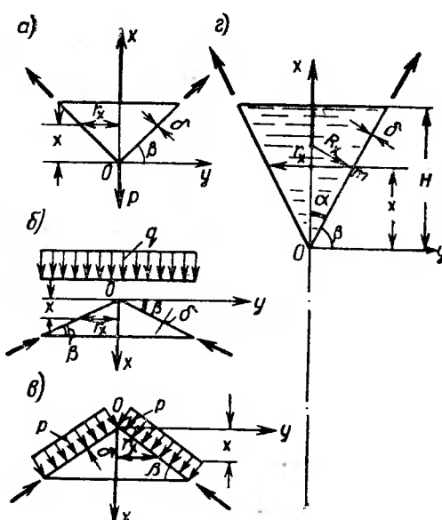
Рис. 17.10. Расчетные схемы для определения напряжений и перемещений безмоментного состояния конических оболочек при различных нагружениях
