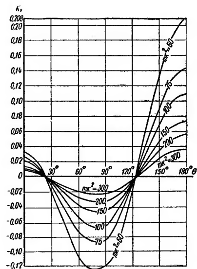
Рис. 3.47. Графики коэффициентов k_1 для определения продольных нормальных усилий N_l от наружного обледенения резервуара
