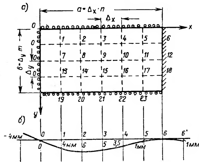
Рис. 16.5. Расчетная схема пластинки, шарнирно опертой по трем сторонам и защемленной по четвертой стороне а — общий вид; б — линия прогиба по оси 1—6
