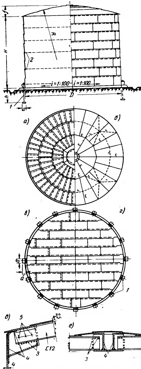
Рис. 3.82. Вертикальный цилиндрический резервуар повышенного давления (РПД) с полусферической каркасной кровлей
