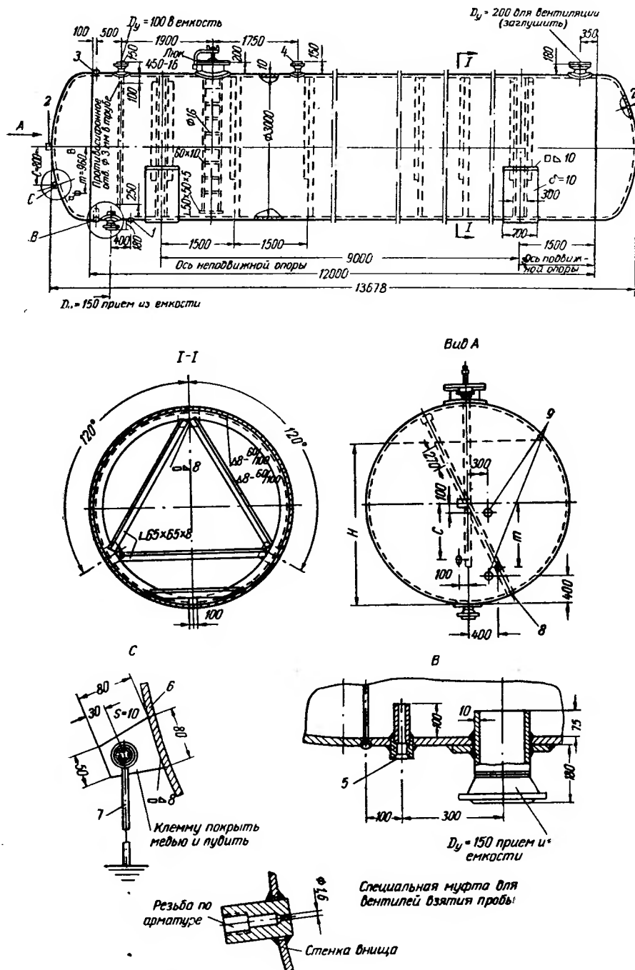
Рис. 3.32. Горизонтальный резервуар с эллипсондальными днищами для легких фракций бензина емкостью 100 м 3
