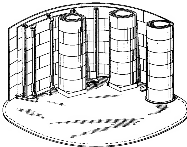
Рис. 12.16. Параллельное разворачивание рулонов
