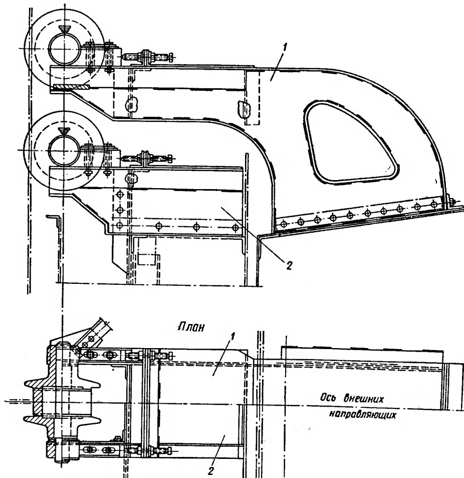
Рис. 6.9. Узлы присоединения внешних роликов мокрого газгольдера 1 — верхний ролик колокола; 2 — верхний ролик телескопа
