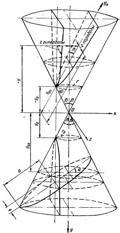
Рис. 2.5. Пересечение конуса плоскостью под углом \leq \beta
