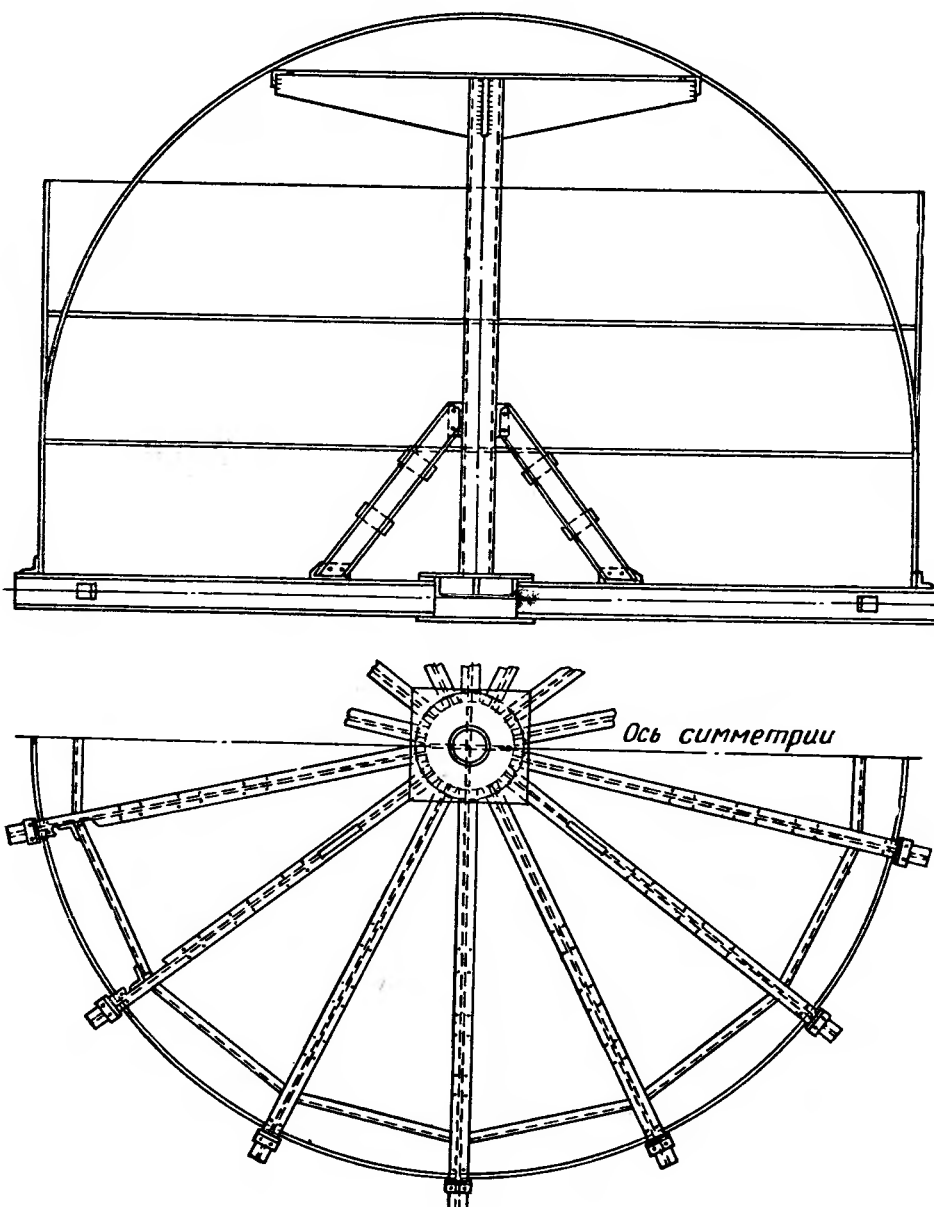
Рис. 11.15. Стенд для сборки обечаек и сферических днищ
