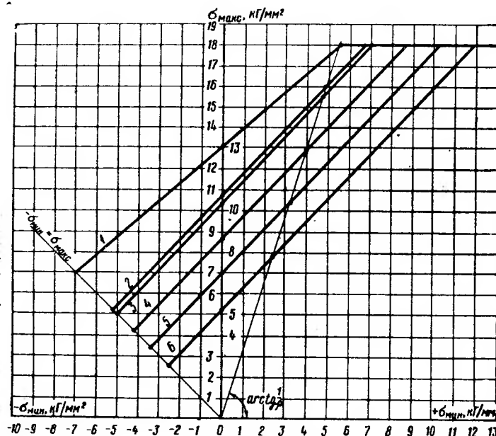
Рис. 21.3. Диаграмма изменения средних значений пределов усталости ( \sigma_{\max} ) основных типов необработанных сварных соединений из углеродистых и низколегированных сталей в зависимости от величины минимальных напряжений цикла.
