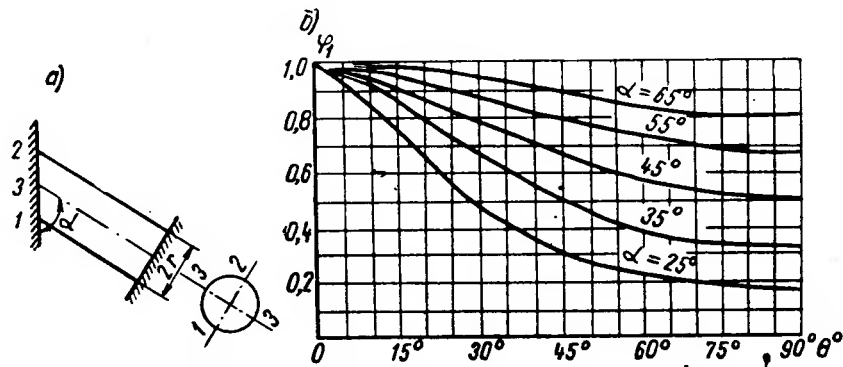
Рис. 9.7. Данные для определения местных напряжений трубы, защемленной по контуру
