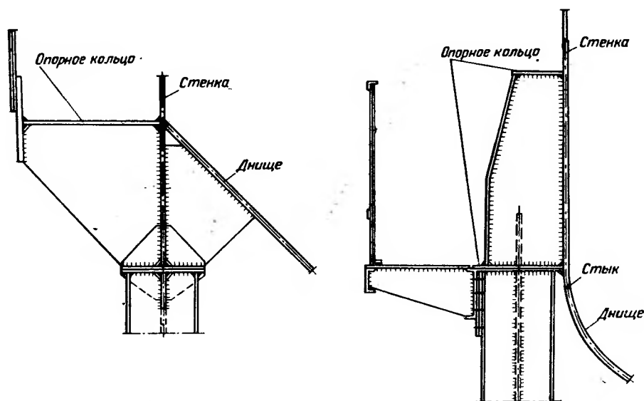
Рис. 4.9. Типы сечений опорных колец резервуаров с пространственным днищем
