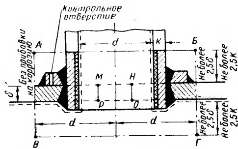
Рис. 5.3. Конструктивное оформление усиления отверстия
