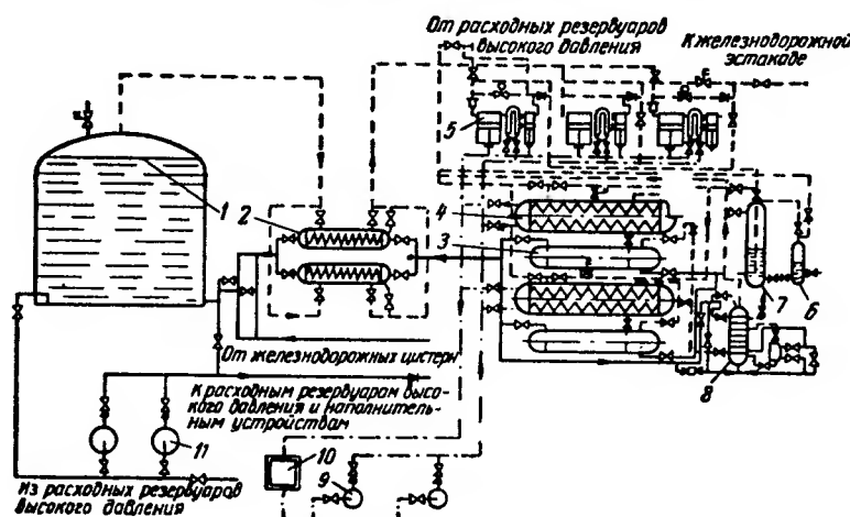
Рис. 3.83. Технологическая схема изотермического хранения сжиженного газа
