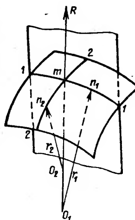
Рис. 17.2. Схема построения главных направлений кривизны и главные радиусы кривизны
