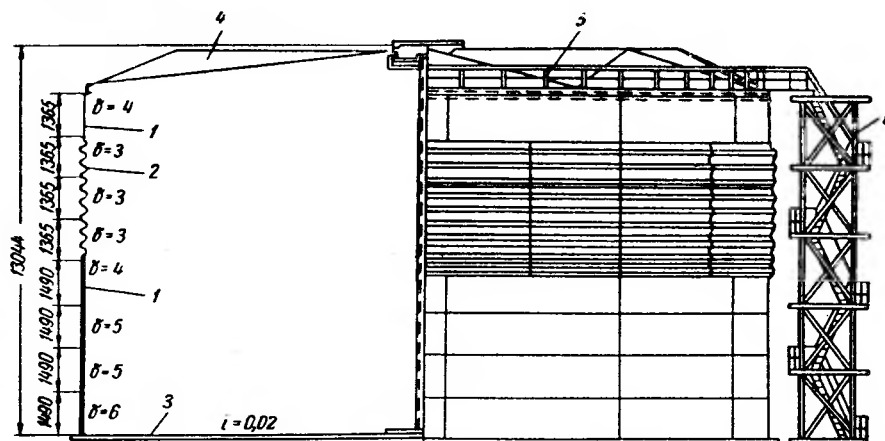
Рис. 3.16. Опытный резервуар емкостью 5000 м³
