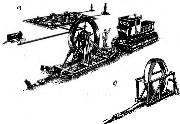
Рис 13.5. Развертывание рулона плоскостворачиваемых труб
