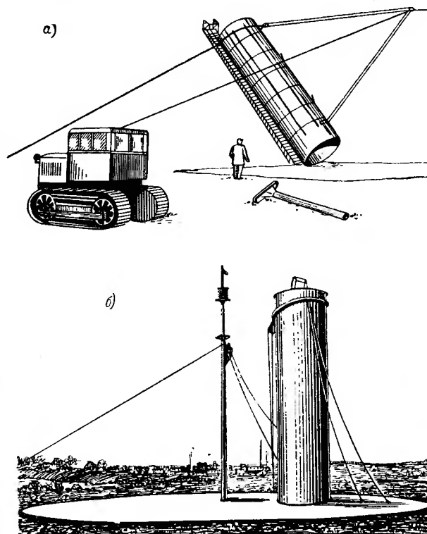
Рис. 12.6. Подъем рулона
