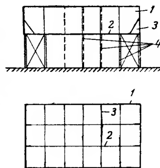
Рис. 10.4. Схема резервуара из плоских щитов
