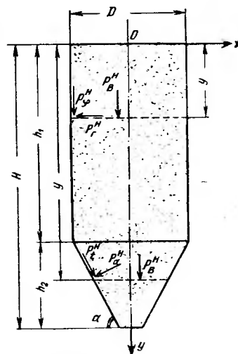
Рис. 7.11. Схема силоса с нагрузками от засыпки
