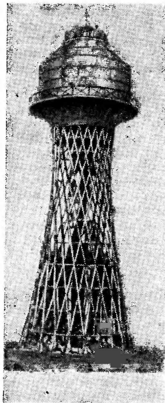
Рис. 1.10. Водонапорная башня системы В. Г. Шухова
