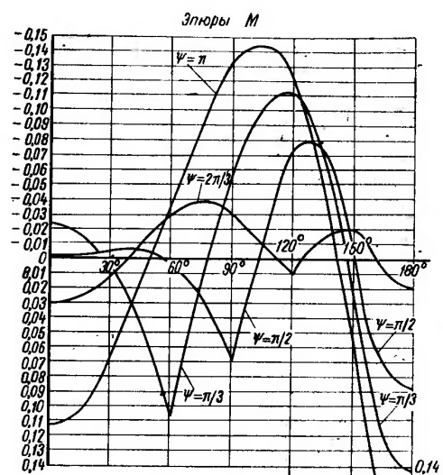
Рис. 3.58. Эпюры M и N в кольце, подкрепленном горизонтальным стержнем и опирающемся на седловую опору с углом охвата 90^\circ
