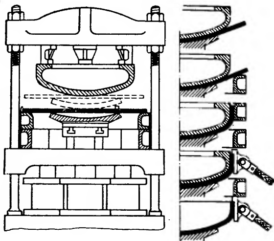
Рис. 11.9. Схема штамповки сферического отбортованного дна на четырехколонном гидравлическом прессе
