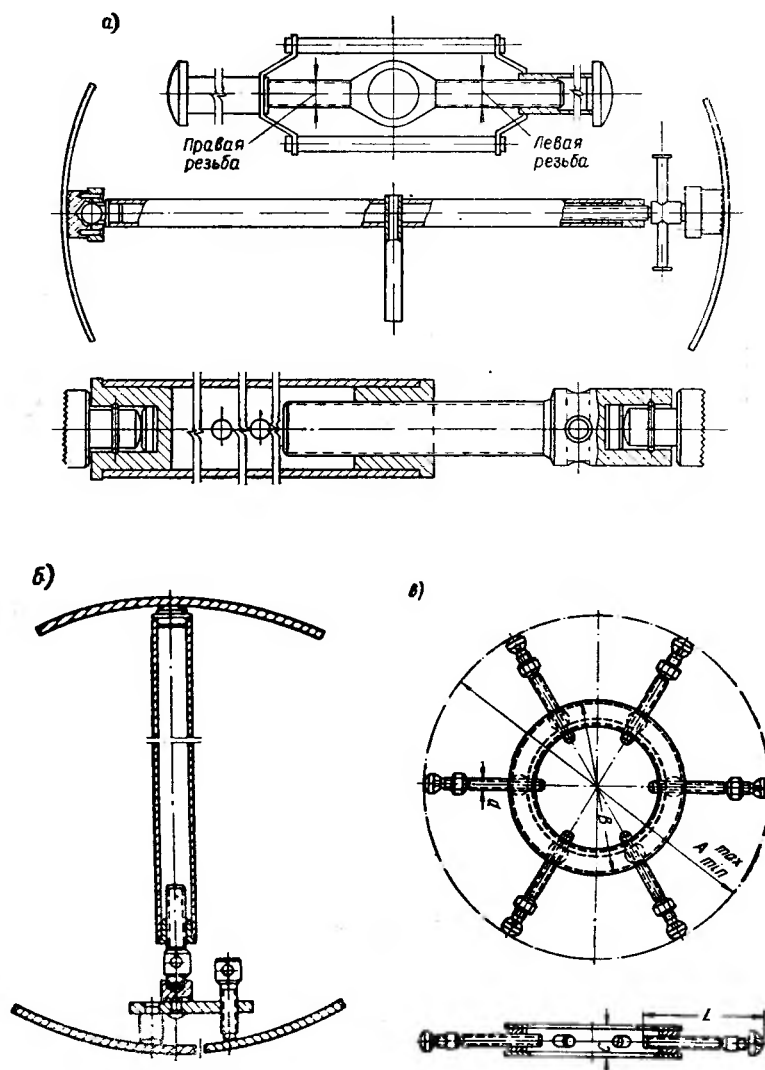
Рис. 11.12. Сборочные распорные приспособления
