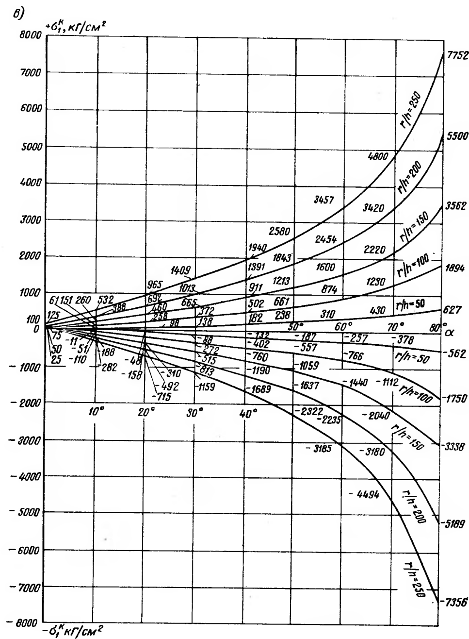
Рис. 19.10, в, г. Графики краевых напряжений при неограниченной упругости в месте пещерах от 10 до 80°; значения r/h ; в — меридиональные напряжения в конической оболочке \sigma_1^k .
