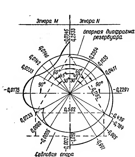
Рис. 3.62. Эпюры M и N в кольце, подкрепленном треугольником и опирающемся на седловую опору с углом охвата 120^\circ
