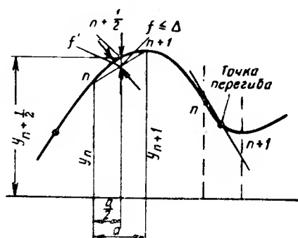
Рис. 2.17. Теоретическая кривая раз- вертки листовой конструкции
