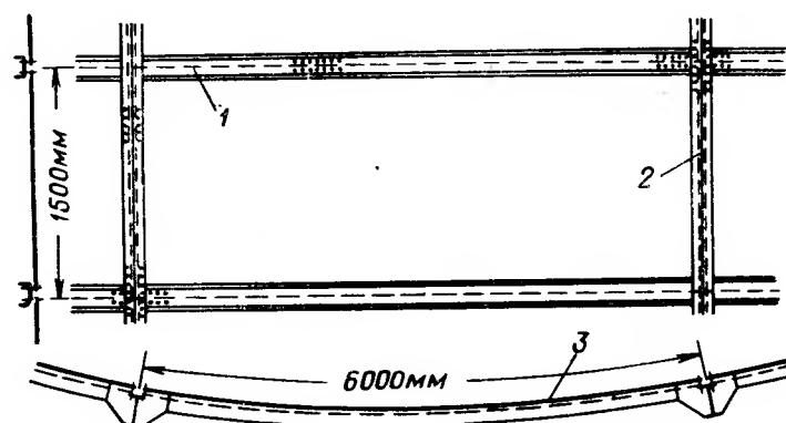
Рис. 6.16. Конструкция стенок сухого газгольдера в клепаном варианте
