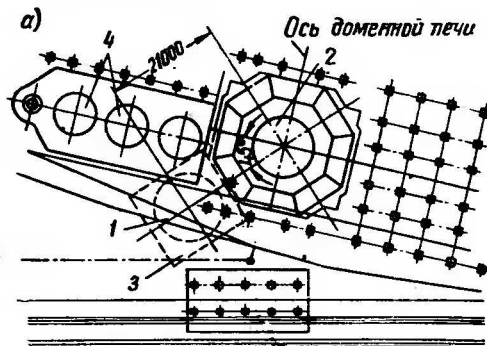
Рис. 12.24. Размещение стенда для реконструкции доменной печи
