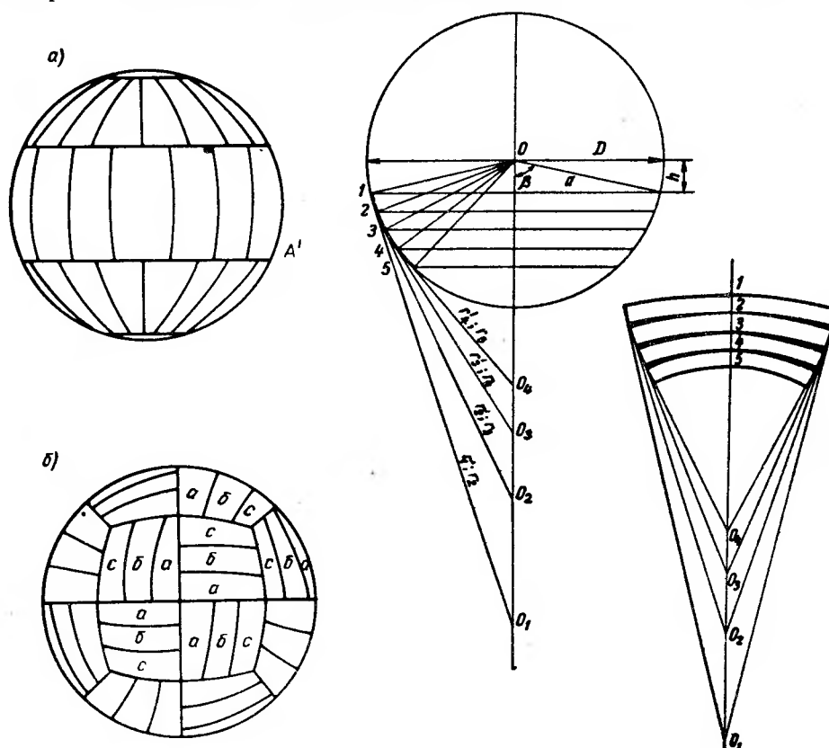
Рис. 2.6. Два способа раскроя поверхности шара
