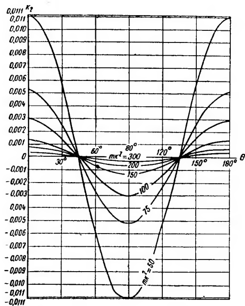
Рис. 3.48. Графики коэффициентов k_2 для определения кольцевых моментов M_2 от наружного обледенения
