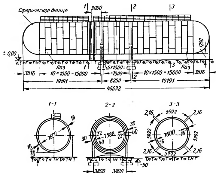
Рис. 5.7. Горизонтальный газгольдер емкостью 2000 \text{ м}^3 , предназначенный для эксплуатации при давлении 4,5 \text{ кг/см}^2
