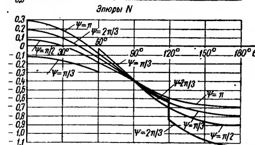
Рис. 3.57. Эпюры M , Q и N в кольце, подкрепленном горизонтальным стержнем и опирающемся на седловую опору с углом охвата 120^\circ
