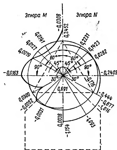
Рис. 3.63. Эпюры M и N в кольце, подкрепленном треугольником и опирающемся на седловую опору с углом охвата 90^\circ
