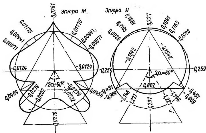
Рис. 3.64. Эпюры M и N в кольце, подкрепленном треугольником и опирающемся на седловую опору с углом охвата 60^\circ
