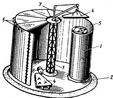
Рис. 12.7. Последовательность монтажа рулонного резервуара с щитовой кровлей
