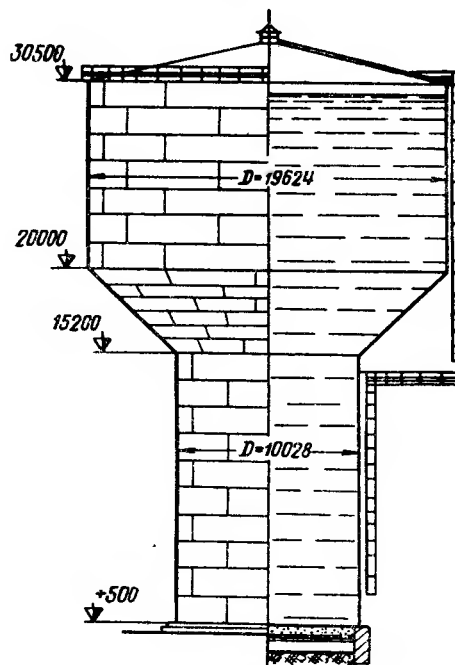
Рис. 4.8. Бесстоечная водонапорная башня емкостью 3000 м³
