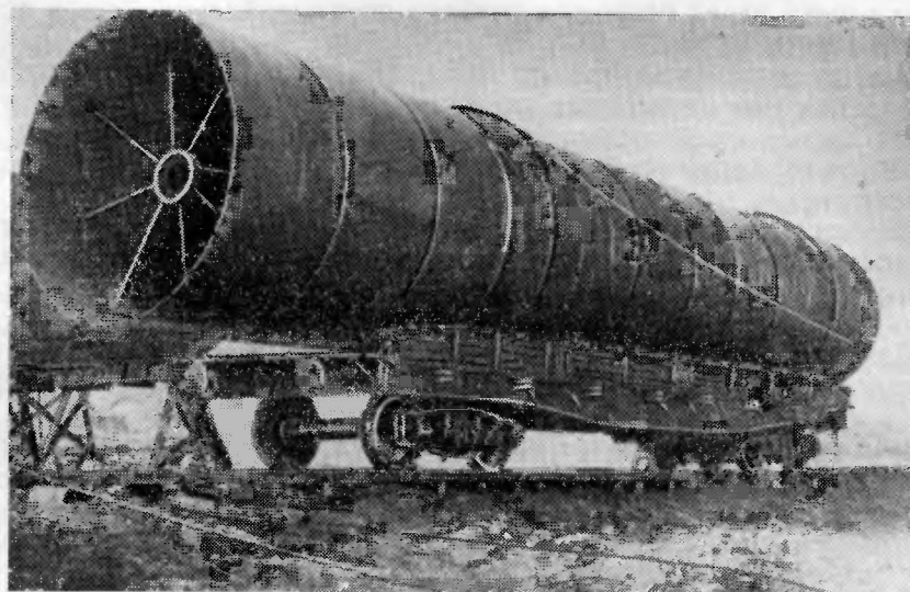
Рис. 12.5. Приспособление для сохранения формы гибкой цилиндрической царги
