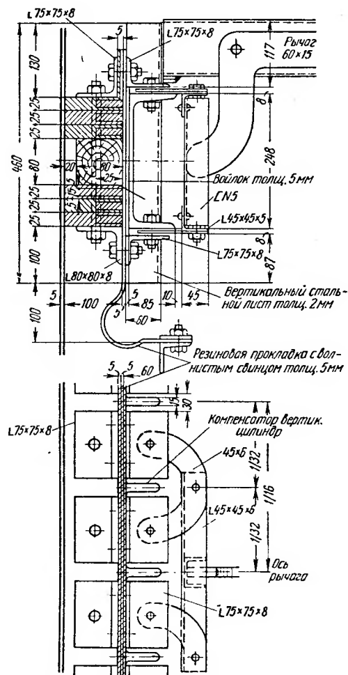
Рис. 6.15. Деталь уплотнения затвора сухого газгольдера с консистентной смазкой
