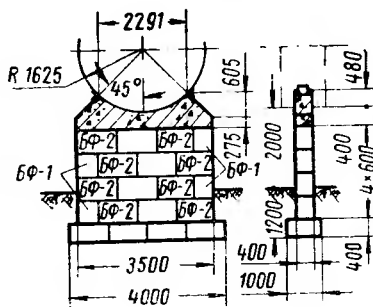
Рис. 3.34. Седловая опора из бетонных блоков высотой 2 м для резервуара емкостью 75 м³ с углом охвата 90°
