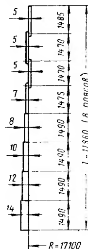
Рис. 3.21. Сечение корпуса резервуара емкостью 10 000 м³
