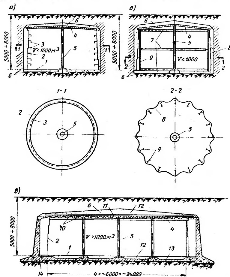
Рис. 3.87. Типы подземных вертикальных цилиндрических резервуаров а — бесказематный резервуар с жесткой оболочкой, усиленной кольцами жесткости; б — бесказематный резервуар с гибкой оболочкой на каркасе; в — резервуар в каземате; 1 — стальное днище; 2 — стенка корпуса; 3 — кольца жесткости; 4 — покрытие; 5 — стальные стойки; 6 — гидроизоляция и антикоррозионное покрытие; 7 — горизонтальные кольца каркаса; 8 — гибкая оболочка корпуса; 9 — стойки каркаса корпуса; 10 — балочная клетка покрытия; 11 — стальная изоляция толщиной 2,5 мм; 12 — гидрофобный песок; 13 — железобетонное днище каземата; 14 — стенки каземата
