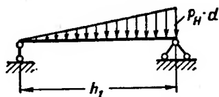
Рис. 7.7. Расчетная схема полочки, вырезанной из стенки бункера
