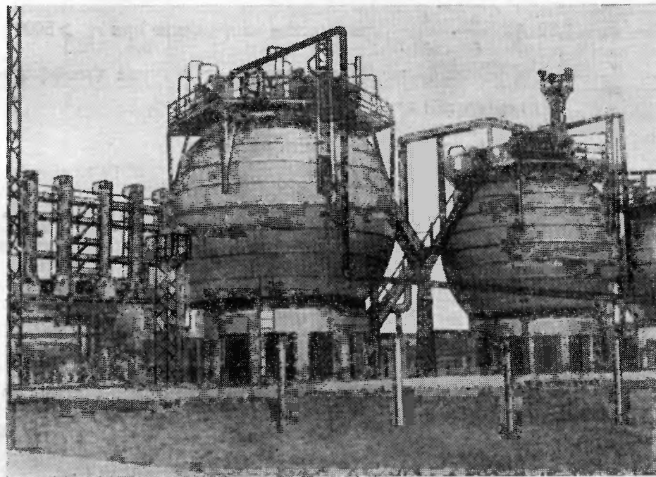
Рис. 3.71. Шаровые резервуары на нефтехимическом комбинате
