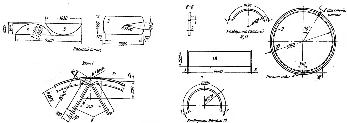
Рис. 3.30. Типовой горизонтальный резервуар емкостью 75 м 3 с пологими коническими днищами 1-18 — номера деталей
