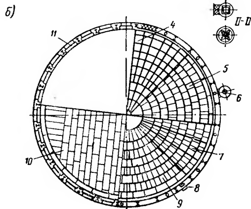
а — вертикальный разрез; б — план; 1 — площадка фонаря; 2 — цепная лестница; 3 — подъемная лестница; 4 — стропила поршня; 5 — настил поршня; 6 — подъемник; 7 — стропила крыши; 8 — направляющие цепной лестницы; 9 — настил крыши; 10 — движце; 11 — фундамент
