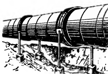
Рис. 1.4. Напорный трубопровод гидроэлектростанции
