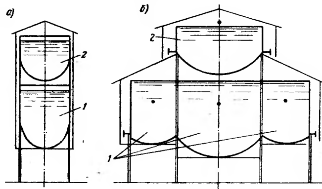
Рис. 10.7. Схема водонапорных башен с двумя резервуарами а — объемом до 1000 м 3 ; б — объемом более 1000 м 3 ; 1 — нижний резервуар; 2 — верхний резервуар
