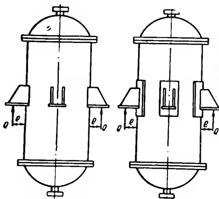
Рис. 4.5. Вертикальные аппараты на подвесных опорах
