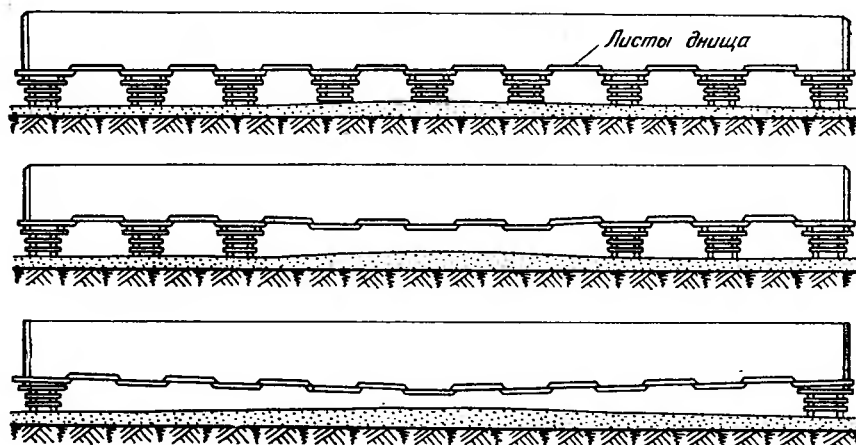
Рис. 12.8. Схема разборки клеток и опускания днища на основание
