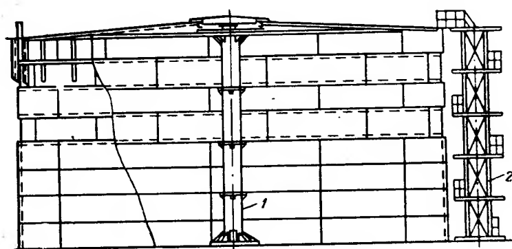
Рис. 3.6. Вертикальный цилиндрический резервуар емкостью 5000 м 3 с центральной стойкой и щитовым покрытием
