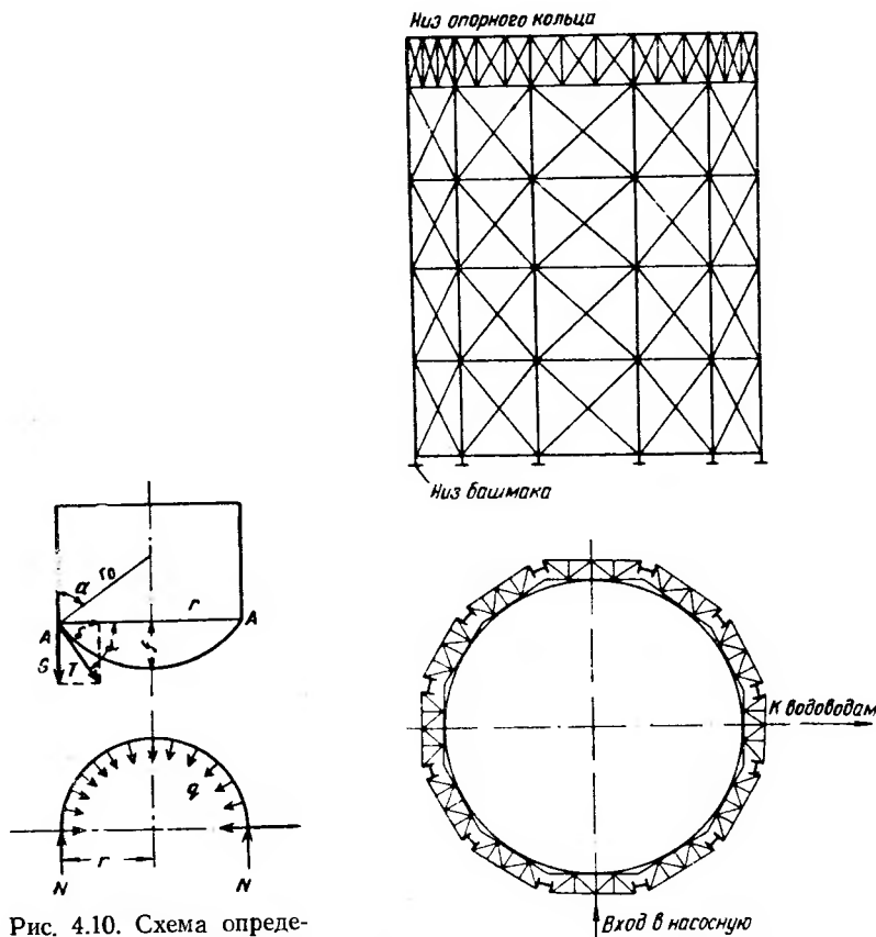
Рис. 4.10. Схема определения сжимающего усилия в опорном кольце резервуара с пространственным дном
