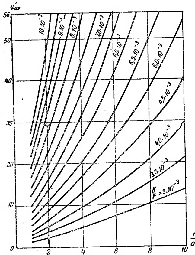
Рис. 18.7. Графики значений q'_{0s} по формуле (18.47) для случая S=0
