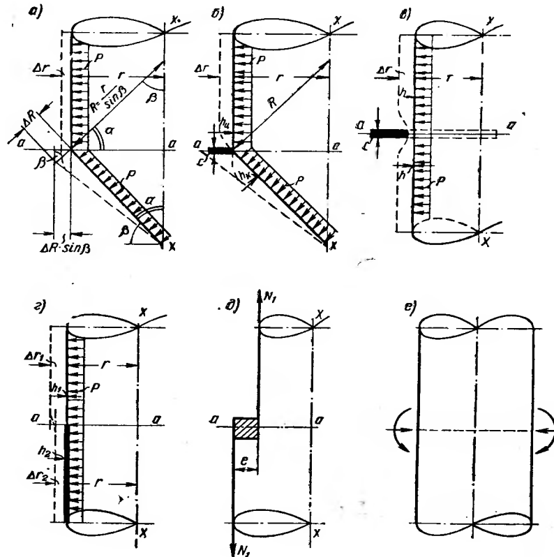
Рис. 19.2. Схемы пересечений оболочек и примыканий к ним
