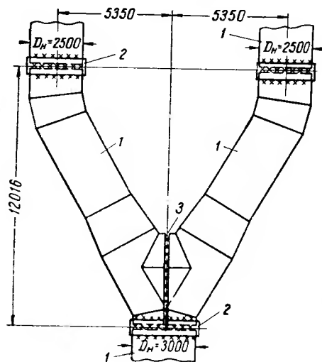
Рис. 12.23. Негабаритный тройник газоотводов
