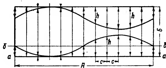
Рис. 11.1. Разметка колена трубопровода на гибком шаблоне; размеры A , B , шаг стрелок c и величины стрелок h даются в рабочем чертеже
