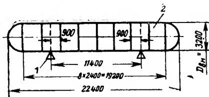
Рис. 3.33. Схема горизонтального резервуара с полушаровыми днищами емкостью 175 м³
