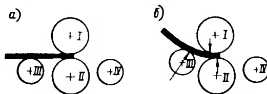
Рис. 11.6. Схема работы четырехвалковых вальцов а — при правке; б — при вальцовке
