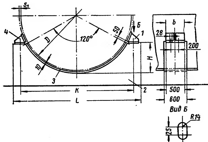
Рис. 3.36. Схема установки резервуара для сжиженных газов на железобетонный постамент с углом охвата 120^\circ
