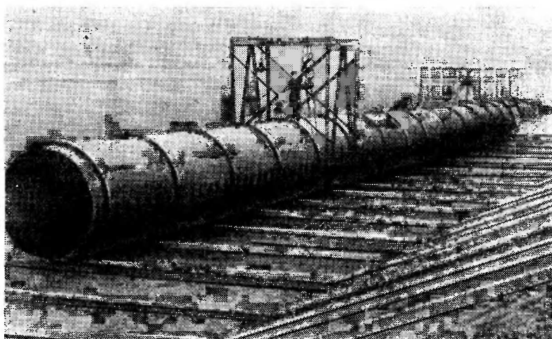
Рис. 12.25. Сборка секций теплофикационного тоннеля на соединительном стеллаже
