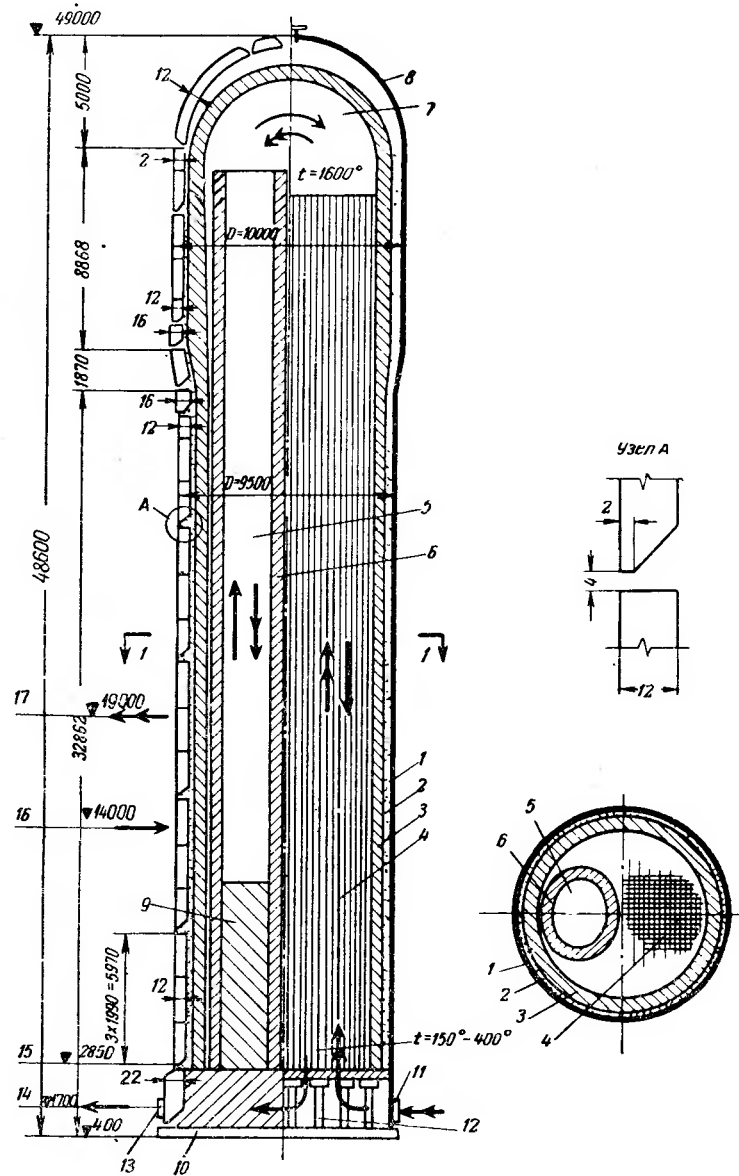
Рис. 8.3. Схема устройства воздухоподогревателя и геометрическая схема кожуха типовой доменной печи объемом 2700 м 3
