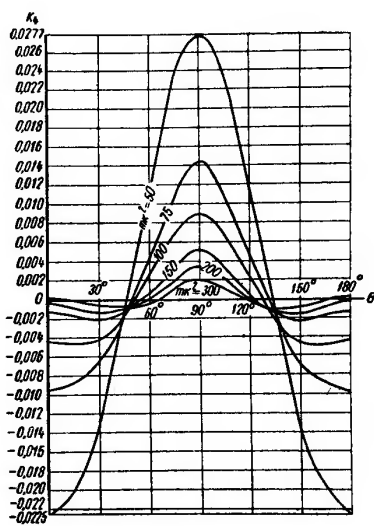
Рис. 3.46. Графики коэффициентов k_4 для определения радиальных перемещений w точек среднего поперечного сечения корпуса от гидростатического давления жидкости, частично заполняющей резервуар
