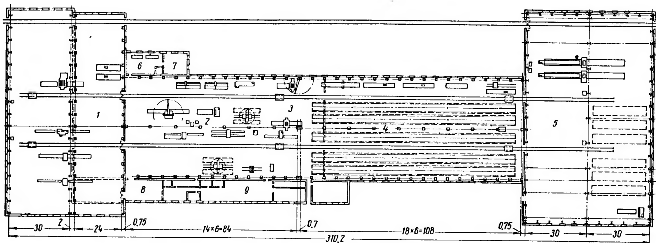
Рис. 11.34. Технологическая схема завода, изготавливающего конструкции малого и среднего веса (трубопроводы, габаритные резервуары и др.), производительностью 20—40 тыс. т в год 1 — цех подготовки; 2 — цех обработки; 3 — склад деталей; 4 — цех сборки; 5 — малярно-погрузочный цех; 6 — разметочная; 7 — ремонтно-строительный цех; 8 — кузнечно-метизный цех; 9 — ремонтно-механический цех
