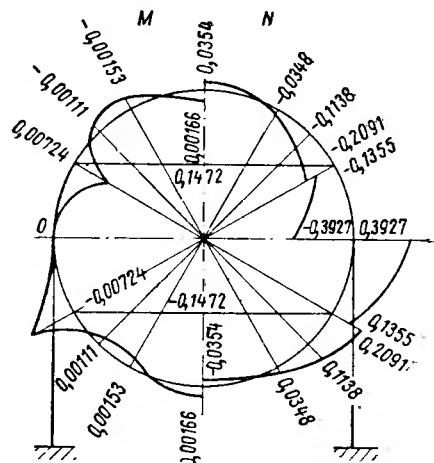
Рис. 3.61. Эпюры M и N в кольце, подкрепленном двумя горизонтальными стержнями и опирающемся на две стойки
