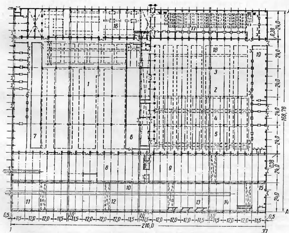
Рис. 11.36. Технологическая схема завода алюминиевых конструкций
