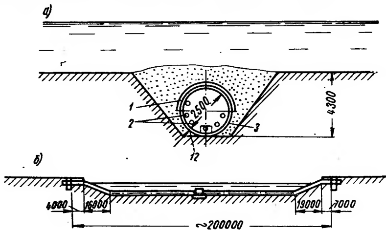
Рис. 9.9. Схема дюкера
