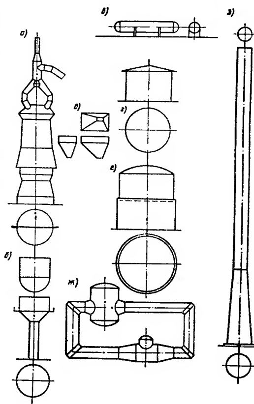
Рис. 2.2. Примеры геометрических форм различных листовых конструкций
