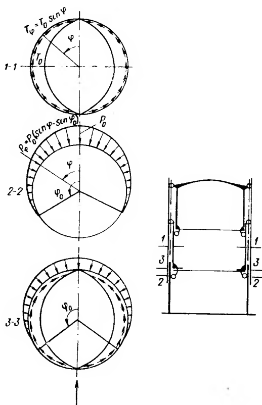
Рис. 6.3. Схема передачи усиления от колокола к телескопу и от телескопа к бассейну
