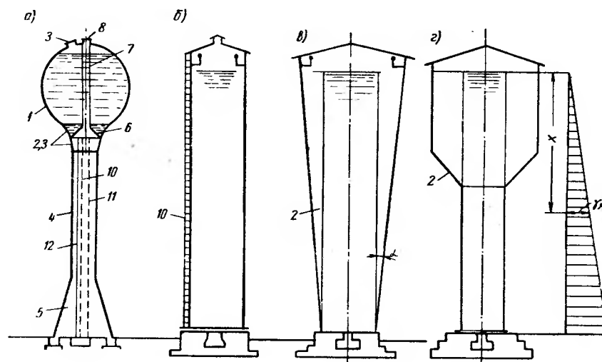
Рис. 10.8. Схемы гидрорезервуаров
