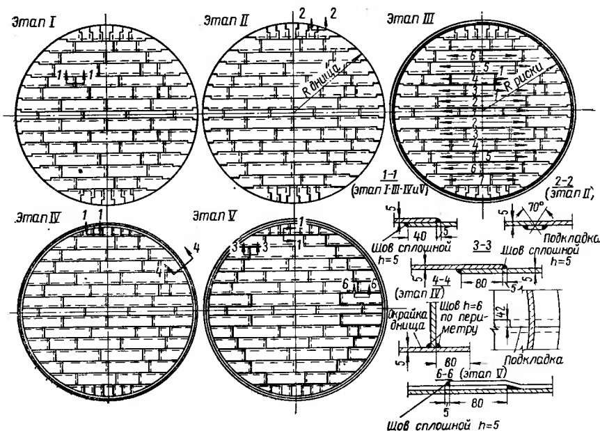
Рис. 12.9. Последовательность монтажа днища цилиндрического резервуара
