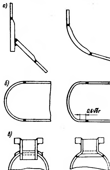
Рис. 21.2. Отбортовка и конические вставки в зоне местных напряжений
