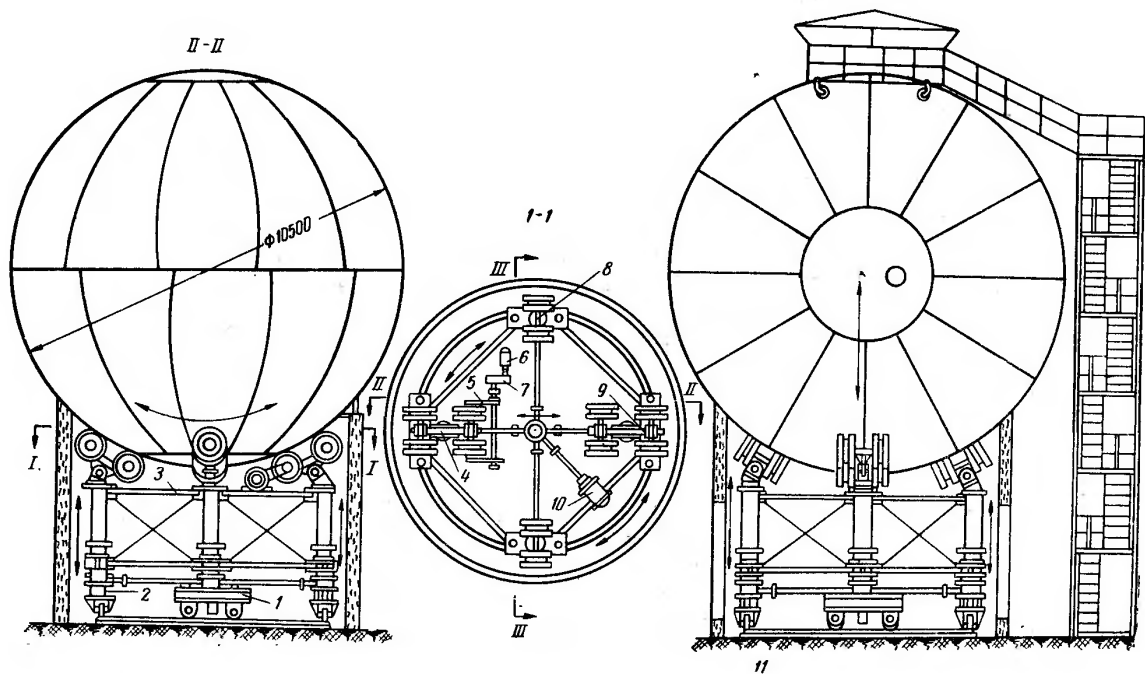
Рис. 3.74. Манипулятор для сварки шаровых резервуаров
