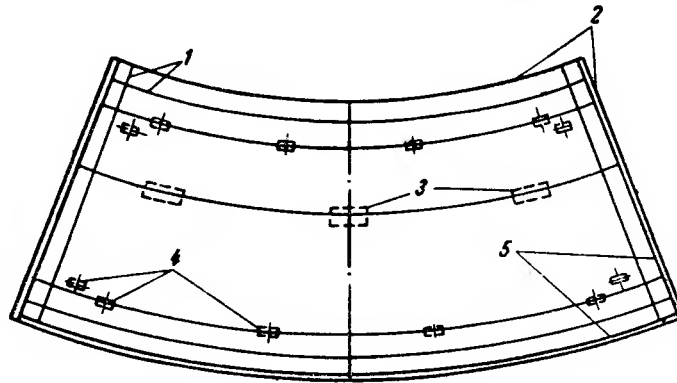
Рис. 11.3. Пример разметки листовой детали кожуха доменной печи
