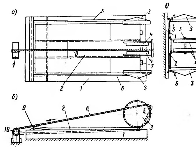
Рис. 11.17. Сборка габаритного резервуара методом наворачивания (Челябинский завод металлоконструкций им. С. Орджоникидзе)
