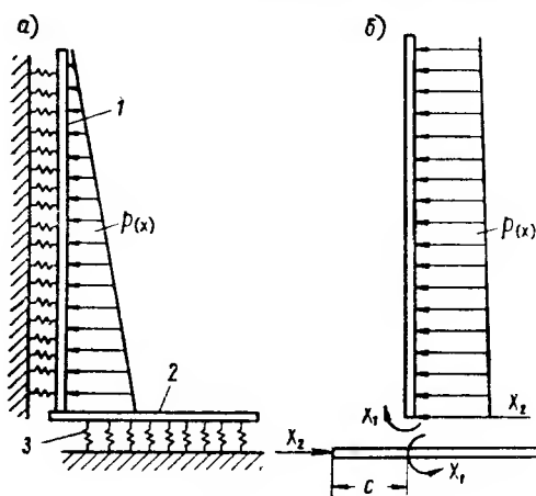
Рис. 3.17. Сопряжение корпуса с днищем
