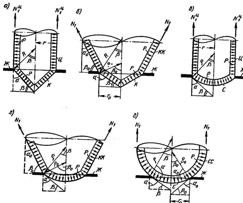
Рис. 19.13. Системы пересечения оболочек с кольцами жесткости
