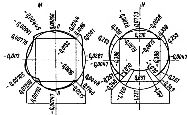
Рис. 3.66. Эпюры M , Q и N в кольце, подкрепленном квадратом и опирающемся на седловую опору с углом охвата 90^\circ
