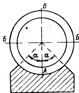
Рис. 9.2. Опираие трубопровода на железобетонную сплошную опору
