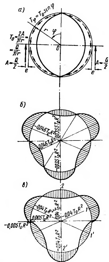
Рис. 5.5. Эпюры моментов у опор горизонтального газгольдера ( Q — нагрузка, приходящаяся на одно кольцо жесткости)
