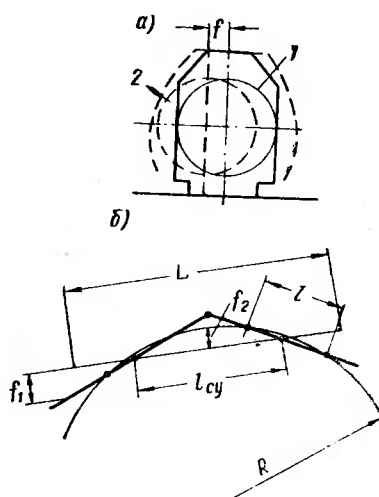
Рис. 13.2. Положение грузов на закруглениях железных дорог
