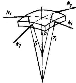
Рис. 3.77. Элемент оболочки каплевидного резервуара двойной кривизны
