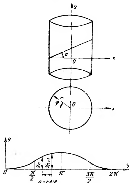
Рис. 2.18. Пересечение цилиндра плоскостью
