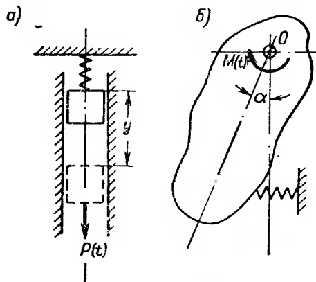
Рис. 16.3. Расчетная схема движения упругой системы с одной степенью свободы а — поступательное движение; б — вращательное движение
