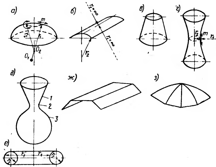
Рис. 17.1. Схемы геометрического построения конструкций оболочек
