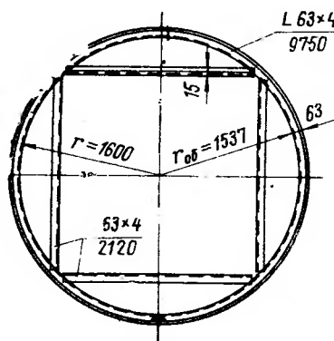
Рис. 3.90. Конструкция диафрагмы заглубленного горизонтального резервуара емкостью 50 \text{ м}^3
