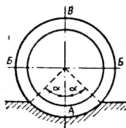
Рис. 9.1. Опираие трубопровода на спрофилированное грунтовое ложе
