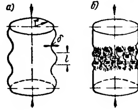
Рис. 18.4. Характерные формы потери устойчивости стенок цилиндрических оболочек при равномерном осевом сжатии
