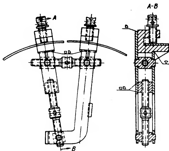
Рис. 11.10. Рычажно-винтовая стяжка
