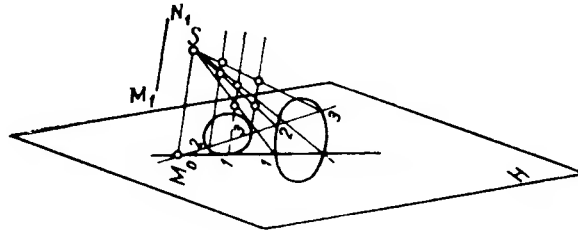
Рис. 2.15. Выбор плоскостей при пересечении конуса с цилиндром
