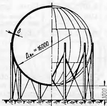
Рис. 3.72. Шаровой резервуар для хранения сжиженного газа, опирающийся на систему стоек
