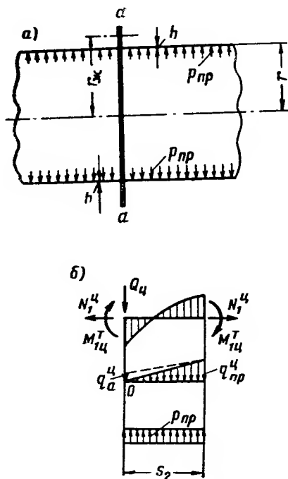
Рис. 19.25. Расчетная схема для определения предельного внутреннего давления p_{\text{пр}} при переходе в пластическую стадию цилиндрической оболочки в зоне примыкания к ней кольца жесткости
