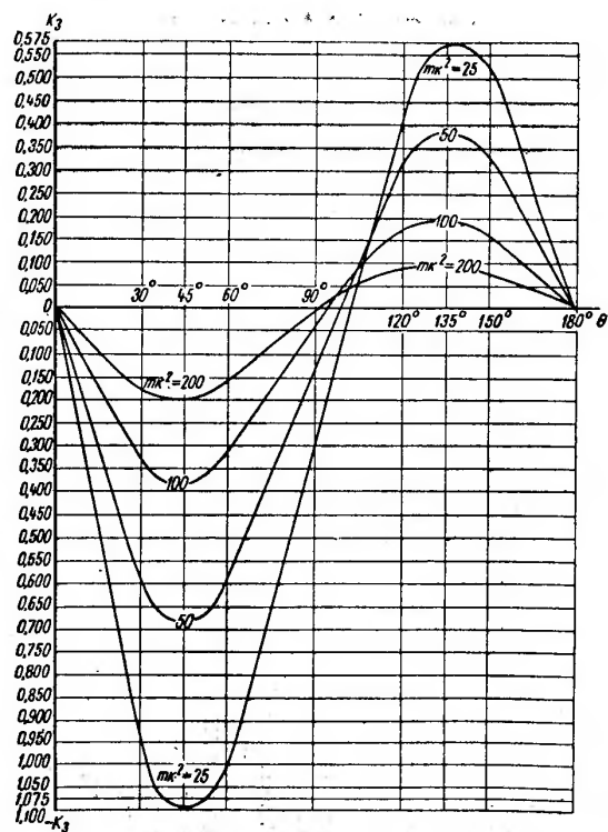
Рис. 3.53. Графики коэффициентов k_3 для определения едвигающих усилий T от ветровой нагрузки
