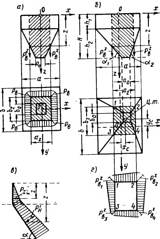
Рис. 7.4. Расчетные схемы бункеров
