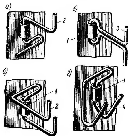
Рис. 1.12. Устройства для крепления наружной тепловой изоляции
