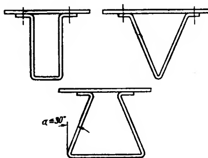
Рис. 14.1. Принципиальное решение конструкций, поддерживающих кровлю, обладающих хорошими антикоррозионными свойствами.
