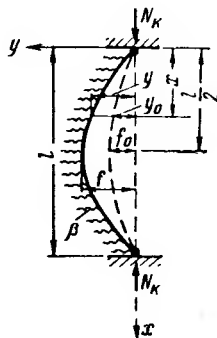
Рис. 18.5. Расчетная схема сжато-изогнутой криволинейной полоски на сплошном упругом основании с начальной стрелкой прогиба f_0
