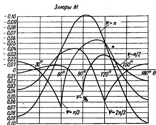
Рис. 3.56. Эпюры моментов и продольных сил в неподкрепленном кольце, опирающемся на седловую опору с углом охвата 2\alpha , равным 180, 120, 90, 60 и 0^\circ (последний случай относится к центральной стойке)
