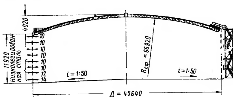
Рис. 3.15. Резервуар емкостью 20 тыс. m^3 со сферической кровлей
