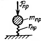
Рис. 16.4. Динамически эквивалентная система с одной степенью свободы P_{пр} — приведенная нагрузка; m_{пр} — приведенная масса; r_{пр} — приведенная жесткость
