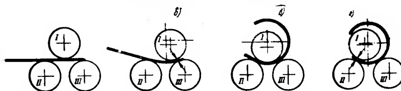
Рис. 11.7. Схема трехвалковых вальцов с подвижным верхним валком в горизонтальной плоскости а — при правке; б — при вальцовке
