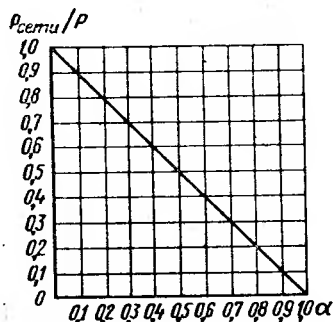
Рис. 5.9. Изменение коэффициента \alpha в зависимости от отношения p_{\text{сети}}/p
