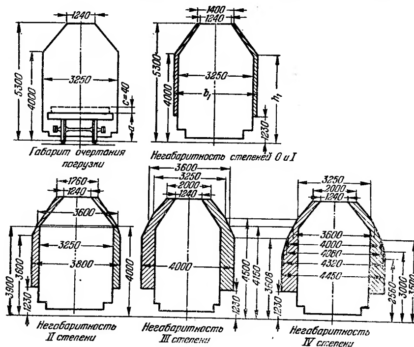
Рис. 13.1. Габарит очертания загрузки
