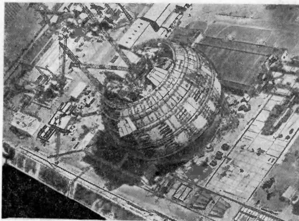
Рис. 12.14. Строительство шарового газгольдера емкостью 87 000 м 3 в г. Шиион (Франция)
