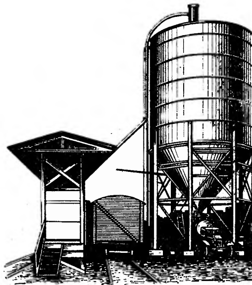
Рис. 7.9. Общий вид круглого бункера
