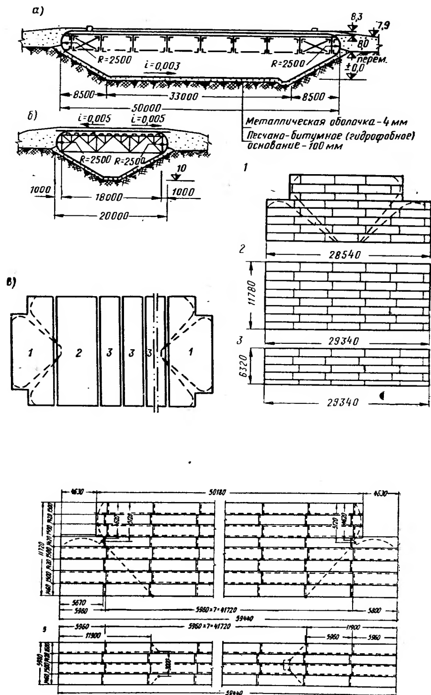
Рис. 3.4. Траншейный резервуар емкостью 5000 м³ с ограждающими стенками в виде стальной оболочки и стальными несущими фермами покрытия а — продольный разрез; б — поперечный разрез; в — развертка оболочки с поперечным раскроем полотнищ; 1 — торцовое полотнище; 2, 3 — поперечные полотнища; 4, 5 — полотнища при продольном раскрое оболочки
