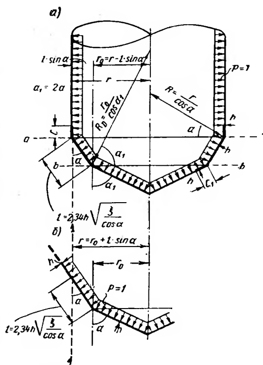
Рис. 19.9. Схемы перехода от конуса к цилиндру через коническую вставку
