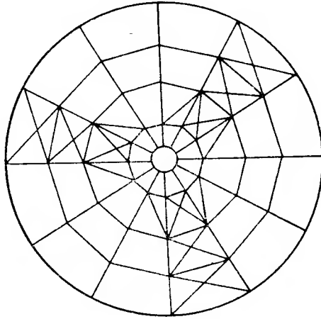
Рис. 6.7. Схема связей при арочном решении кровли
