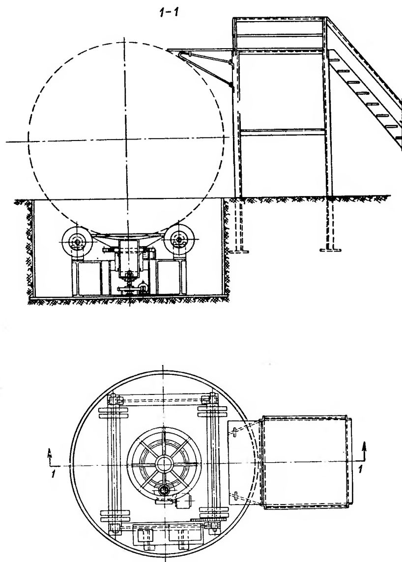
Рис. 11.29. Роликовый стейд для автоматической сварки полушаровых днищ
