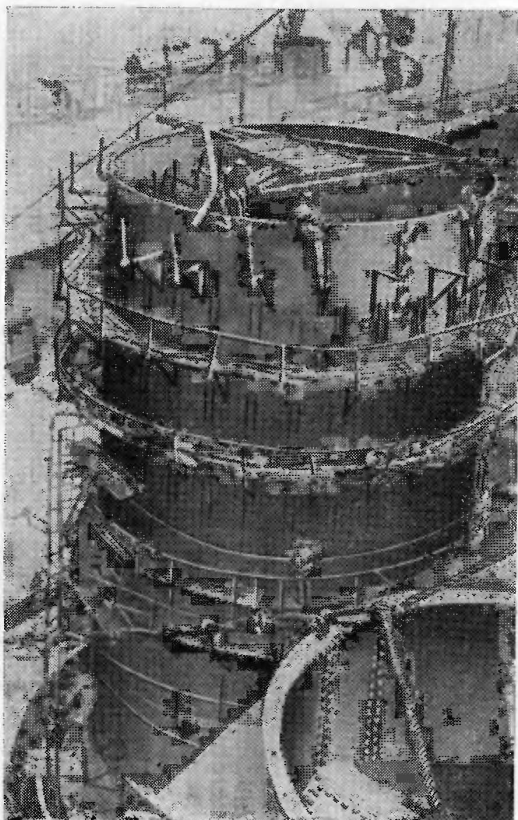
Рис. 12.2. Расположение подмостей при монтаже доменной печи (период до 1960 г.)
