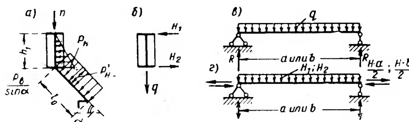
Рис. 7.6. Расчетная схема бункерной балки
