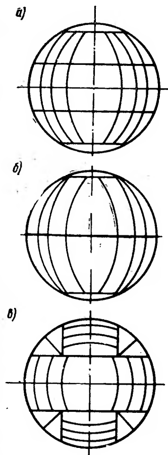
Рис. 3.73. Варианты раскроя шарового резервуара объемом 2000 м 3
