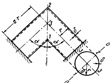
Рис. 9.5. Расчетная схема пересечения двух трубопроводов под произвольным углом (без усиления по линии пересечения)
