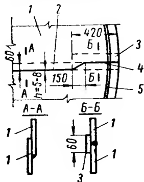
Рис. 3.9. Перевод нахлесточного соединения на стыковое в окрайках днища
