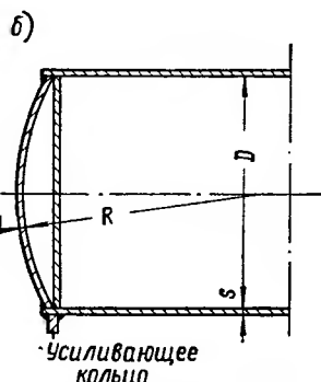
Рис. 3.31. Фрагмент горизонтального резервуара со сферическими неотбортованными днищами
