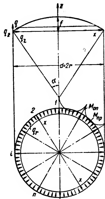
Рис. 6.4. Расчетная схема оболочки колокола и краевого кольца
