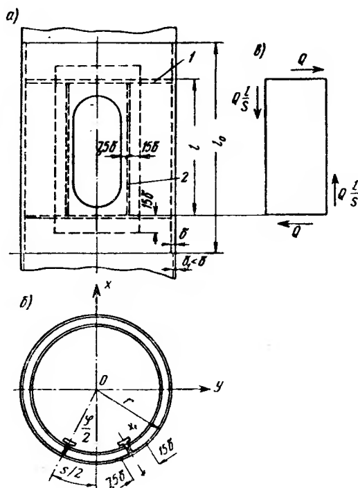
Рис. 10.2. Принципиальная схема укрепления отверстия (выхода) в цилиндрической трубе a — фасад обечайки, имеющей отверстие; b — план; в — схема для расчета зоны укрепления отверстия
