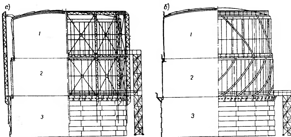
Рис. 1.2. Мокрые газогольдеры
