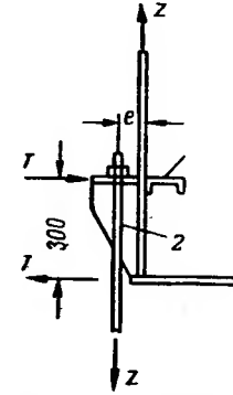
Рис. 3.18. Схема анкерного крепления резервуара
