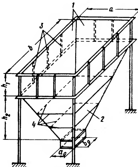
Рис. 7.3. Пространственная схема одноячейкового бункера
