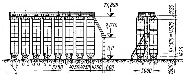
Рис. 5.6. Общий вид батареи из вертикальных газгольдеров 1 — железобетонные сваи или фундаменты
