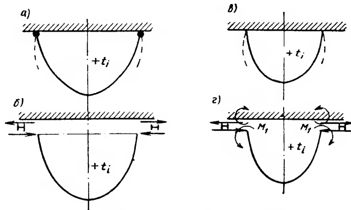
Рис. 20.2. Расчетные схемы для определения краевых усилий от среднего равномерного нагрева по эпюре +t_2
